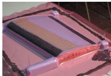
Vakuuma izlīmēšanas process
